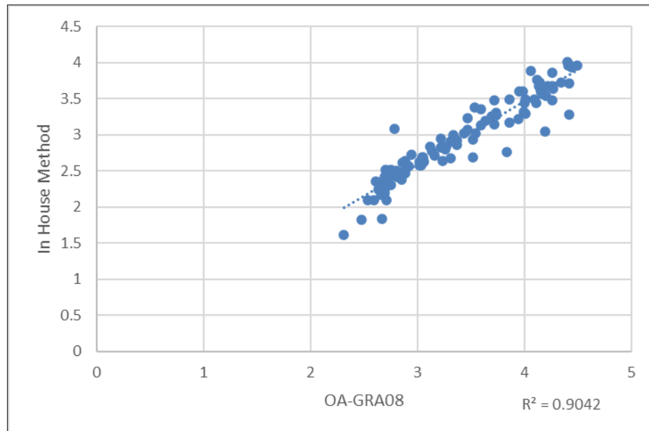
Figure 11.3 Chart comparing ALS method OA-GRA08 with new SFA SG method
