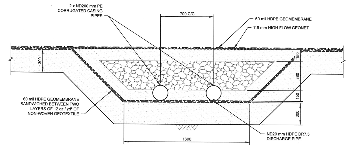
2 SECTION DISCHARGE PIPE TRENCH N.T.S.
